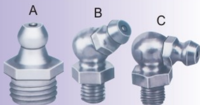
MGM -1209 GREASE NIPPLES A) STRAIGHT B) 45° BENT C) 90° BENT
